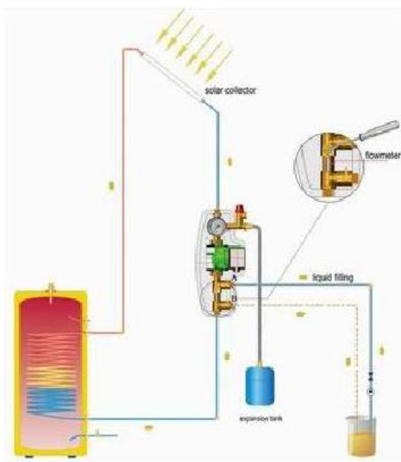
Принципиальная схема солнечной водонагревательной установки под давлением
