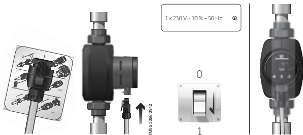
Рис. 12. Подключение к электросети
