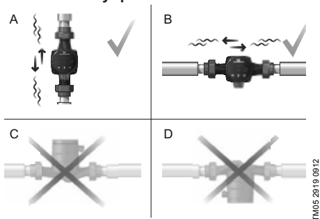
Рис. 6. Положение блока управления
