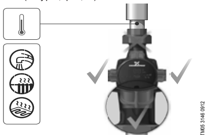
7-сур. Басқару блогының сорғыны жергілікті жылу және ЫСҚЕ жүйелеріне орнату барысындағы орналасуы
