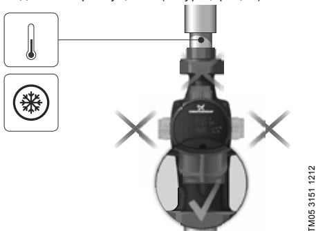
8-сур. Басқару блогының сорғыны жергілікті желдету және ССЖ жүйелеріне орнату барысындағы орналасуы
