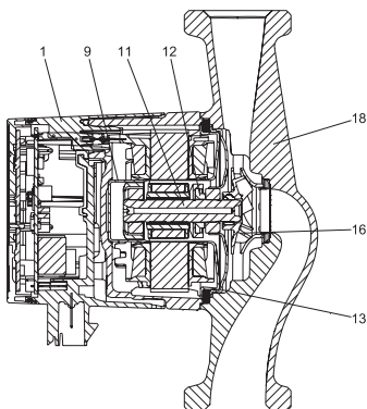
1-сур. ALPHA2 сорғысы кесіндісі
