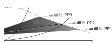
Рис. 19 Три кривые/настройки пропорционального регулирования
