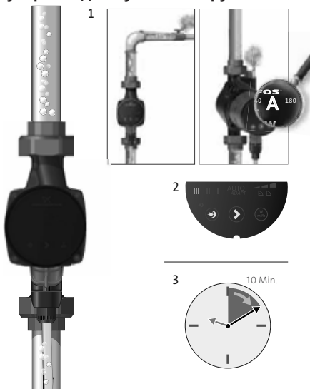
15-сур. Жылу жүйесіндегі ауаны шығару
