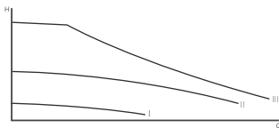
Рис. 24. Выбор настроек насоса в соответствии с типом системы. Заводская настройка: AUTO ADAPT .
