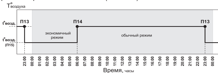
Рис.6 График температуры воздуха в помещении для Режим 2.
