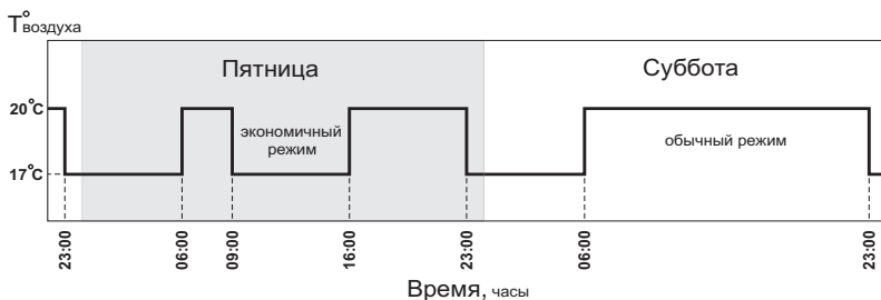
Рис.7 График температуры воздуха в помещении для Режима 3.
