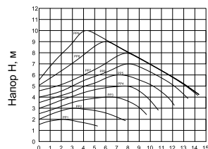
Производительность Q, м³/ч STAR PX1 PP1-PP9
