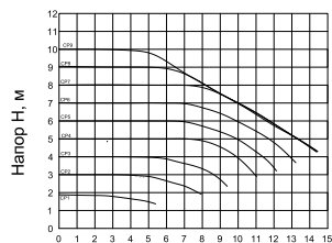
Производительность Q, м³/ч STAR PX1 CP1-CP9
