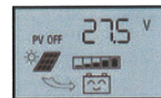
9. Напряжение полного заряда аккумулятора, отключение СБ (программируемый параметр) (LVD)
