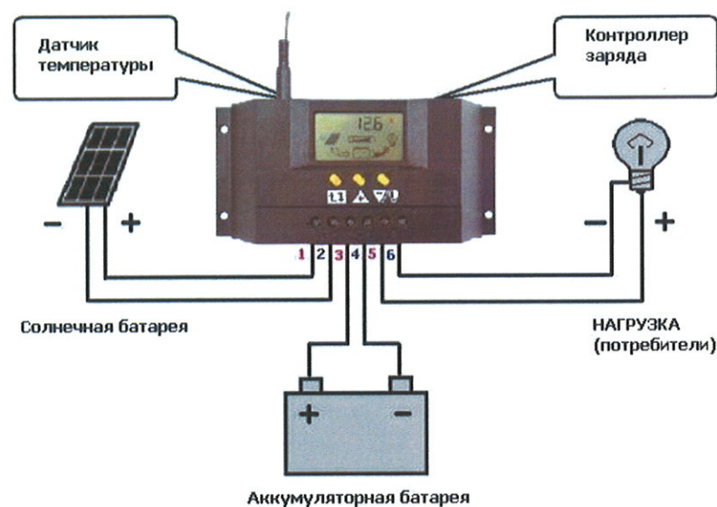
Рисунок 2. подключение контроллера в систему
