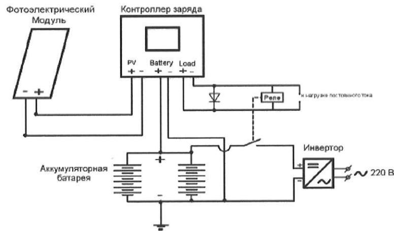
Рисунок 3. Схема подключения инвертора в системе
