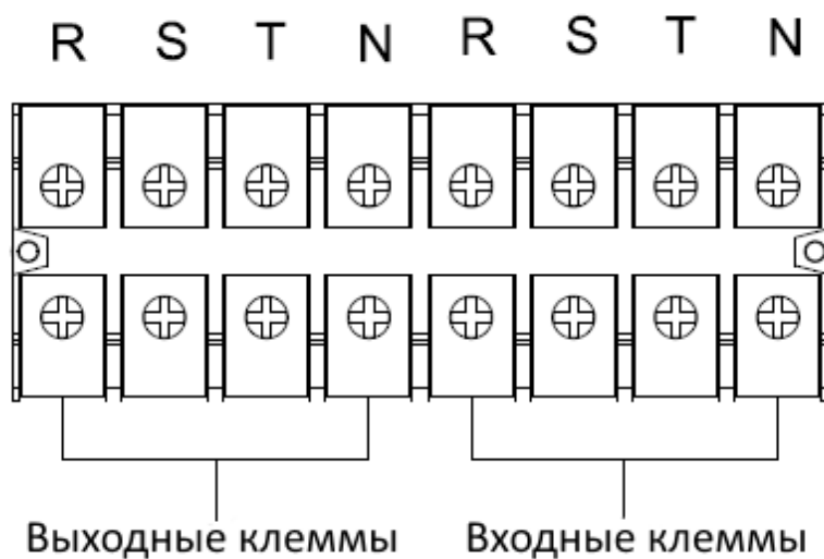
Рис.2-3-2 Блок клемм ИБП G-II 60 / 80 (Long )
