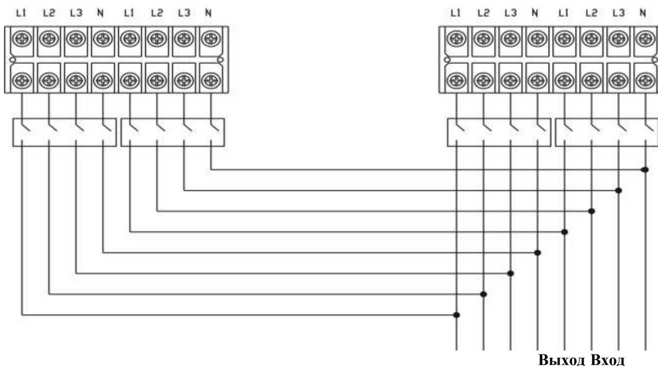
Рис.2-4-1 Подключение в параллельную систему ИБП G-II ( на примере двух ИБП).
