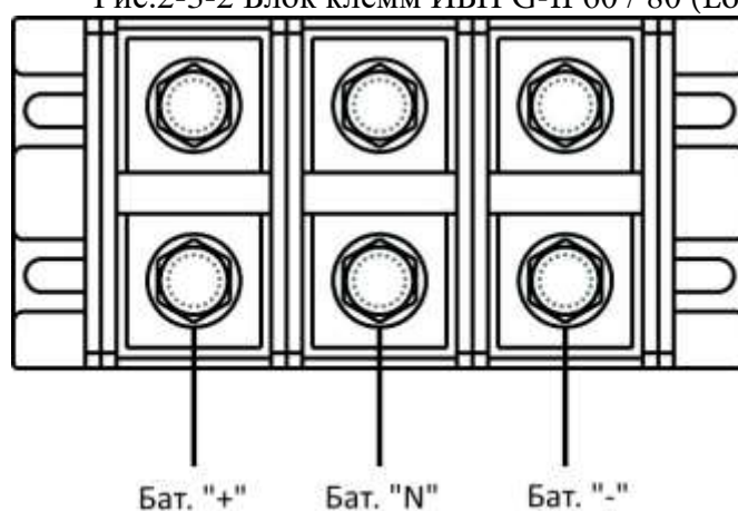
Рис.2-3-3 Блок клемм ИБП G-II 60 / 80 (Long) для подключения аккумуляторных батарей
