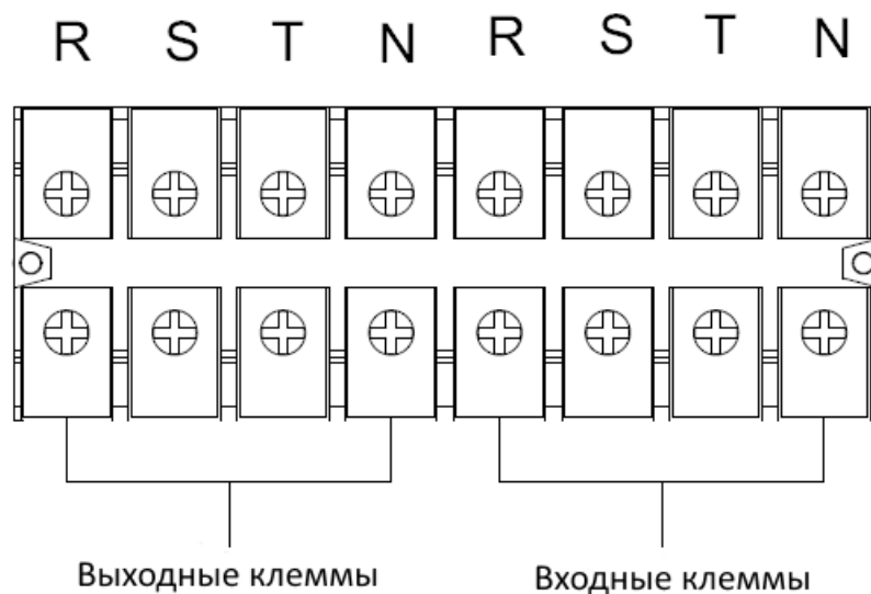
Рис. 2-3-1 Блок клемм ИБП G-II 30 / 40
