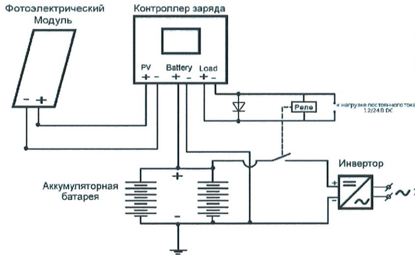
Рисунок 3. Схема подключения инвертора в системе
