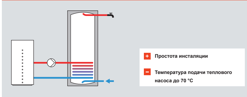
Рис. D.2.1–5 Моновалентный режим нагрева воды
