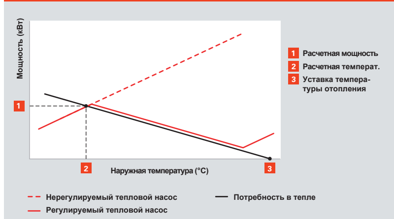
Рис. А.3.1–2 Регулирование мощности
