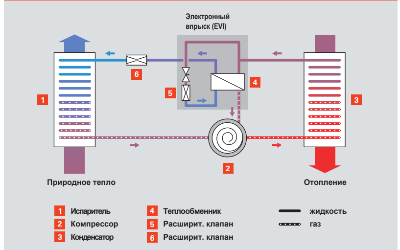
Рис. А.3.1–4 Промежуточный впрыск пара (EVI)
