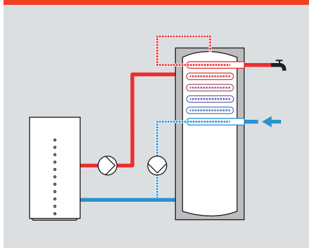
Рис. D.2.1–19 Коаксиальный теплообменник
