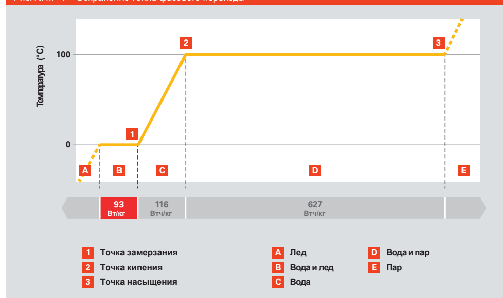
Рис. А.4.7–1 Сохранение тепла фазового перехода
