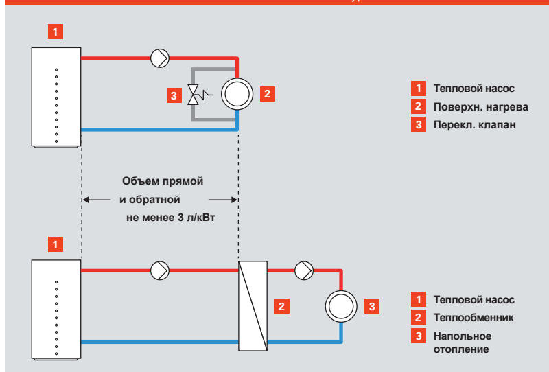
Рис. D.2.2–4 Минимальный объем в отопительном контуре
