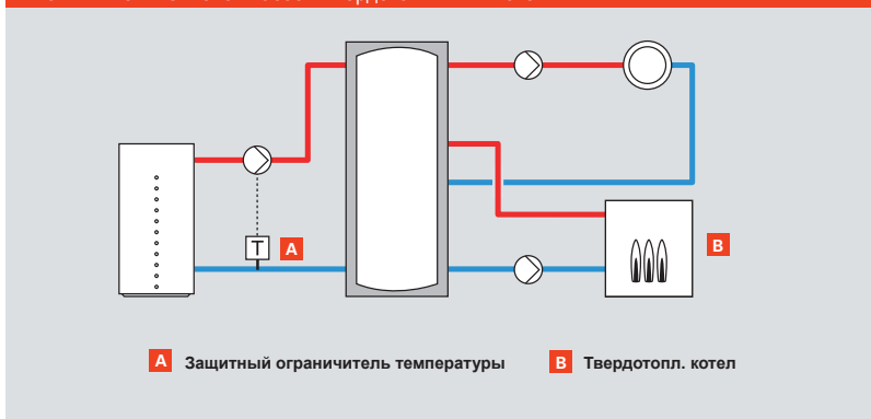
Рис. D.1.4–3 Тепловой насос и твердотопливный котел
