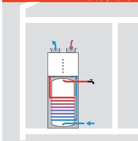
Рис. D.2.1–9 Тепловой насос (с циркуляцией)
