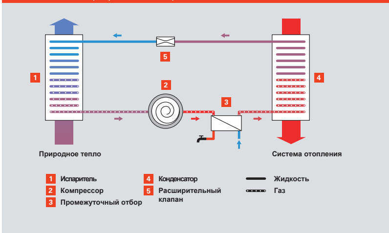
Рис. А.3.3–4 Отбор горячей газовой фазы
