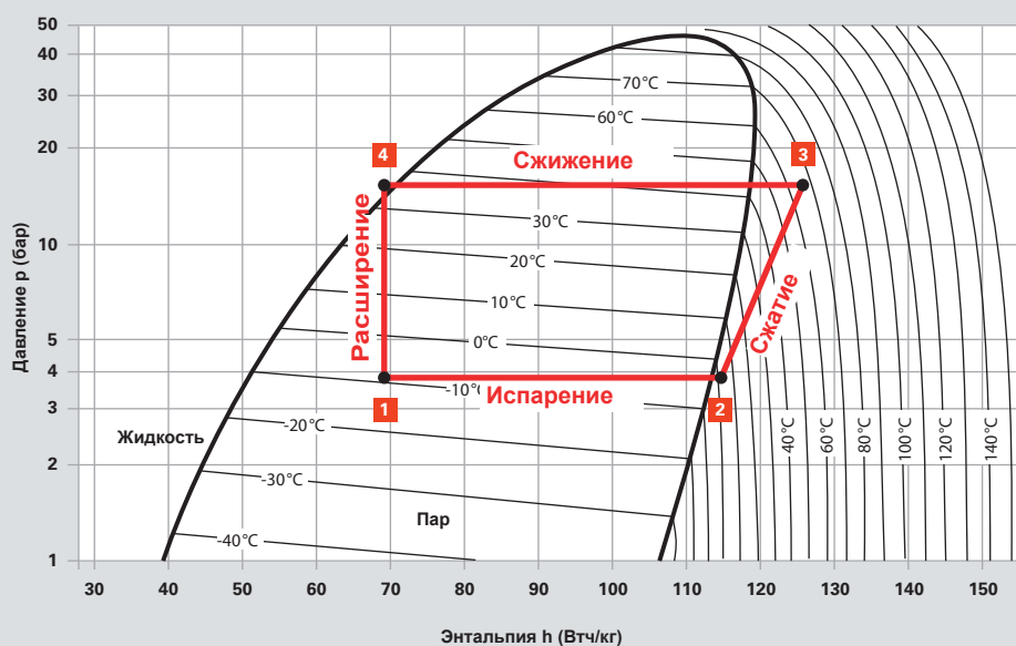
Рис. А.2.2–2 Логарифмическая диаграмма давление/энтальпия
