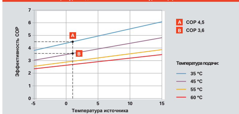
Рис. D.2.2-5 Температура подачи отопительного контура и эффективность
