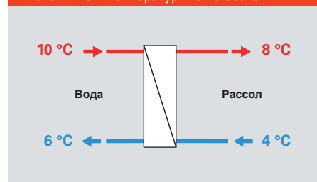
Рис. С.2.1-3 Температурные показатели
