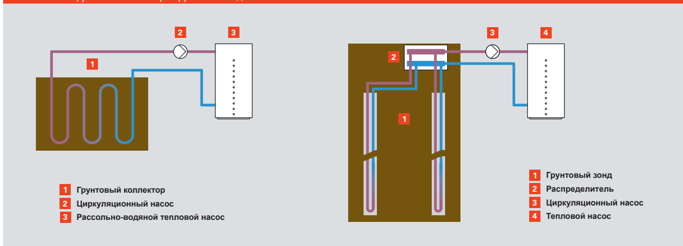
Рис. С.1.1-1 Грунтовый коллектор и грунтовый зонд
