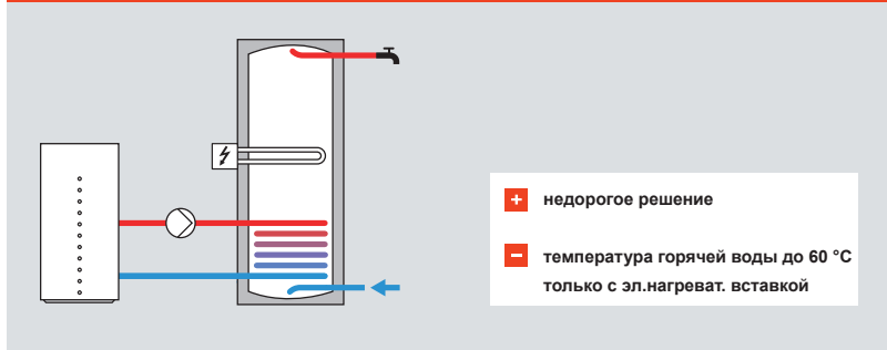
Рис. D.2.1–6 Моноэнергетический режим нагрева воды
