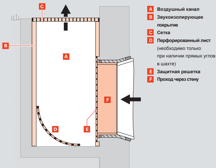
Рис. С.3.4–2 Поток воздуха в канале
