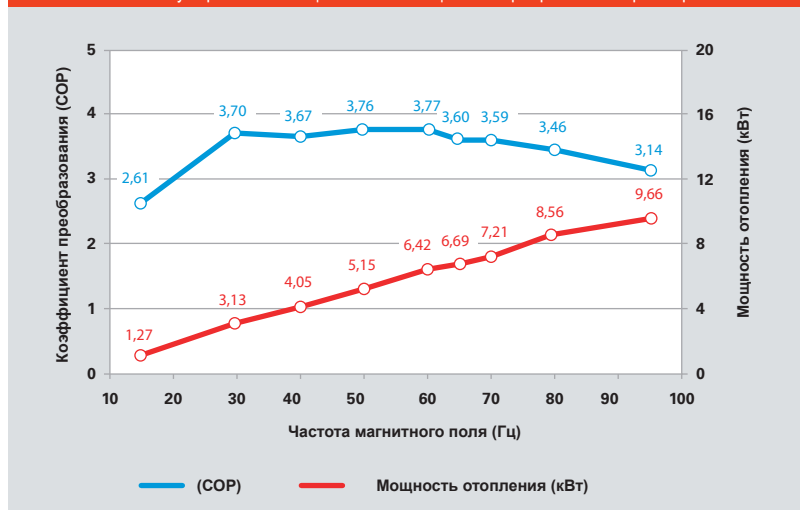
Рис. А.3.1–3 Регулирование мощности с помощью инверторного компрессора
