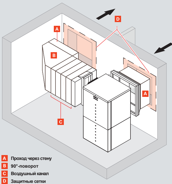
Рис. С.3.4–1 Забор воздуха для внутренней установки
