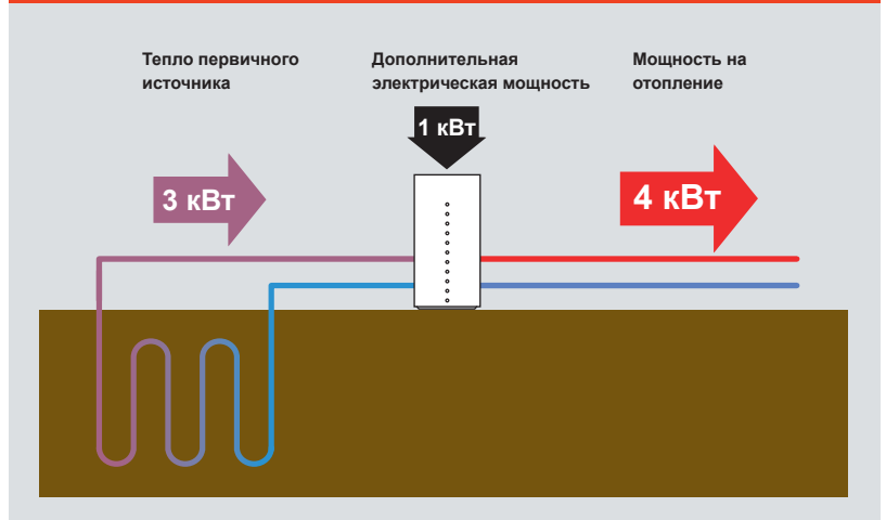
Рис. А.2.3–1 КПД как коэффициент преобразования
