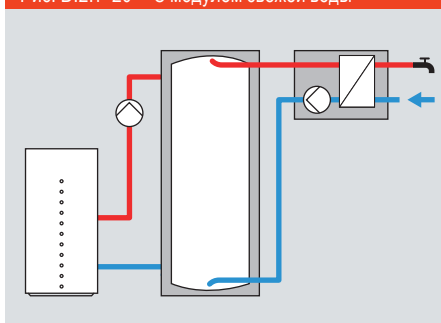
Рис. D.2.1–20 С модулем свежей воды
