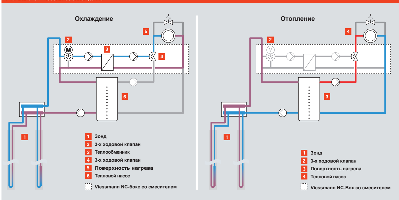
Рис. D.2.3-3 Пассивное охлаждение
