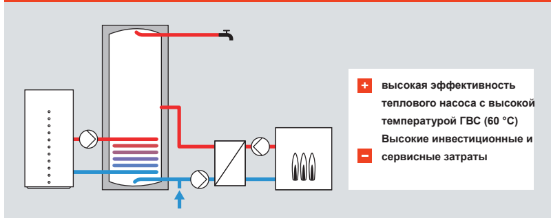
Рис. D.2.1–7 Бивалентный режим
