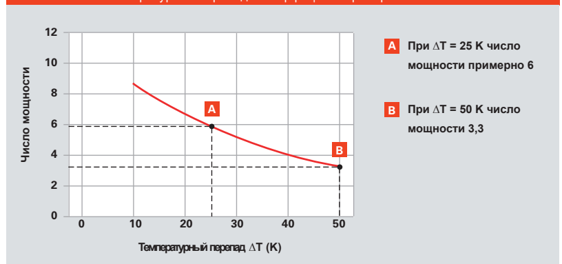
Рис. А.2.3–2 Температурный перепад и коэффициент преобразования
