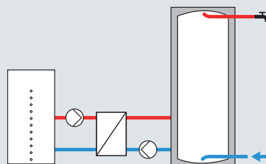
Накопительная емкость с внешним теплообменником
