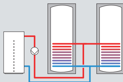
2 параллельно включенных емкости
