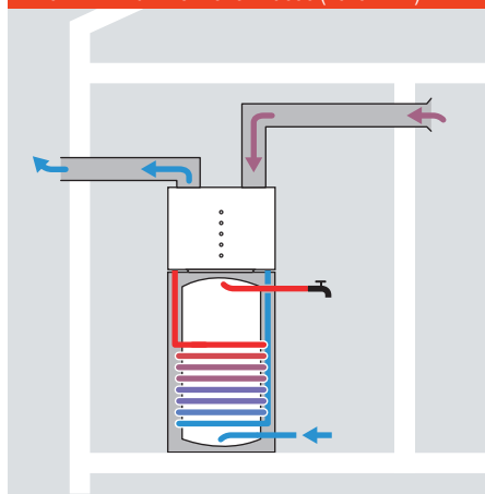
Рис. D.2.1–10 Тепловой насос (поточный)
