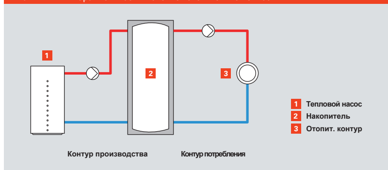
Рис. D.2.2-1 Параллельное включение накопительной емкости
