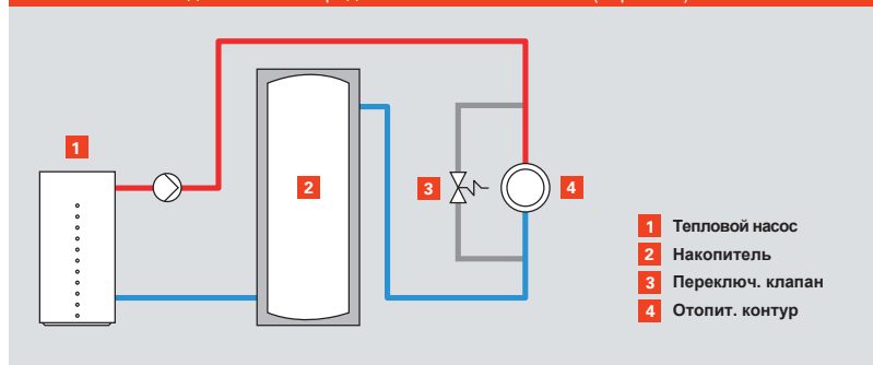
Рис. D.2.2–3 Подключенные в ряд накопительные емкости (обратная)
