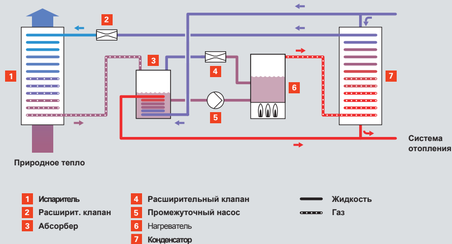
Рис. А.5.2–1 Принципиальная схема работы абсорбционного теплового насоса
