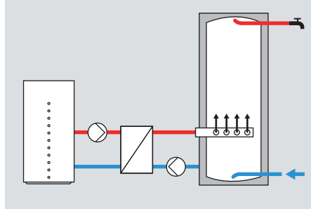
Рис. D.2.1-15 Функциональный принцип
