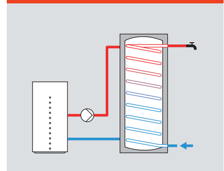
Рис. D.2–18 Змеевиковый теплообменник
