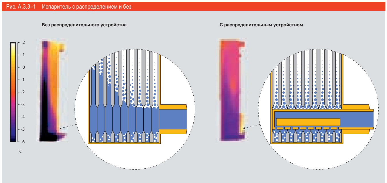
Термографические снимки наглядно показывают распределение тепла в теплообменном аппарате без распределительного устройства (слева), когда хладагент неравномерно покрывает поверхность теплообмена и с распределительным устройством (справа).
