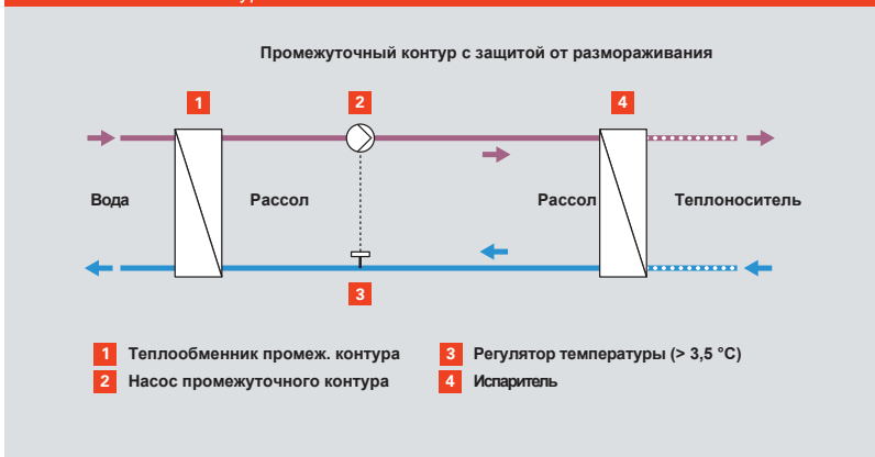
Рис. С.2.1-2 Межконтурный теплообменник
