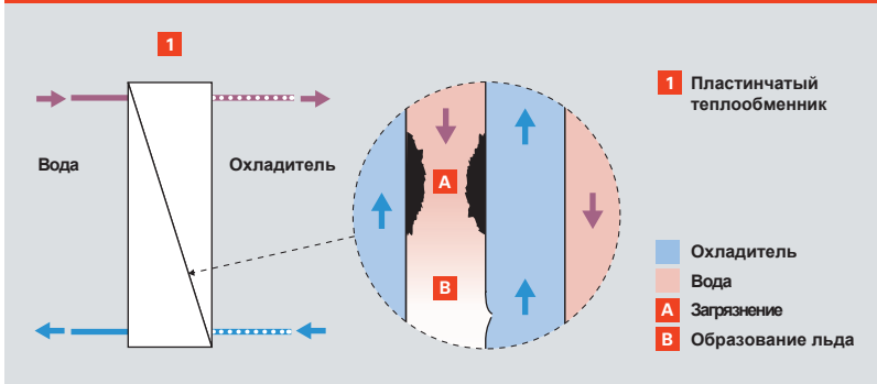
Рис. С.2.1-1 Особенности применения пластинчатого теплообменника
