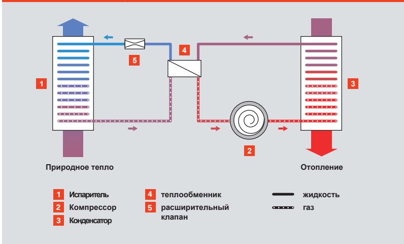
Рис. А.3.3–3 Всасывающий теплообменник
