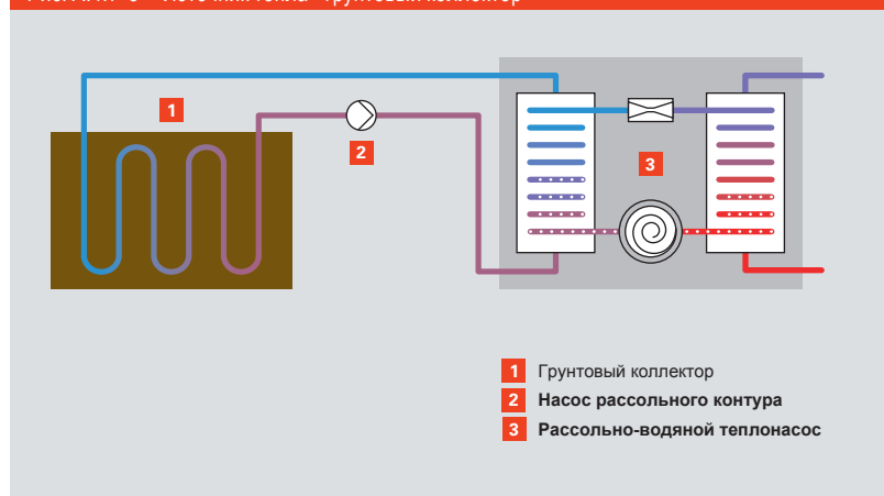
Рис. А.4.1–3 Источник тепла - грунтовый коллектор
