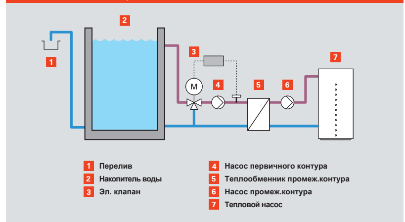
Рис. С.2.2–1 Охлаждающая вода как источник тепла
