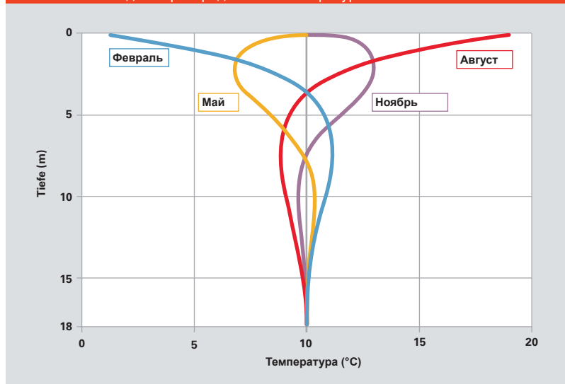
Рис. А.4.1–1 Годовое распределение температуры
