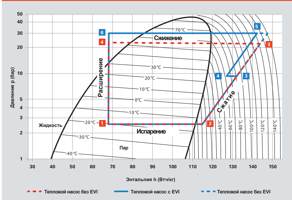
Рис. А.3.1–5 Влияние процесса EVI
