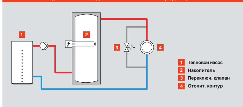
Рис. D.2.2–2 Подключенные в ряд накопительные емкости (подающая)
